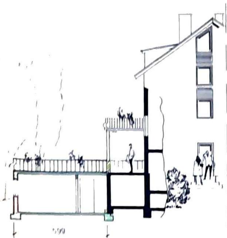
SCHNITT A-A
